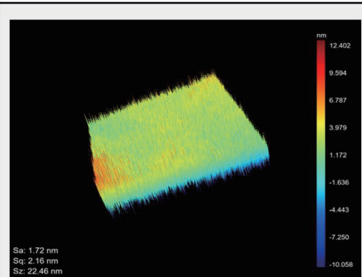
晶圆表面糙度
