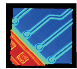
晶圆表面
