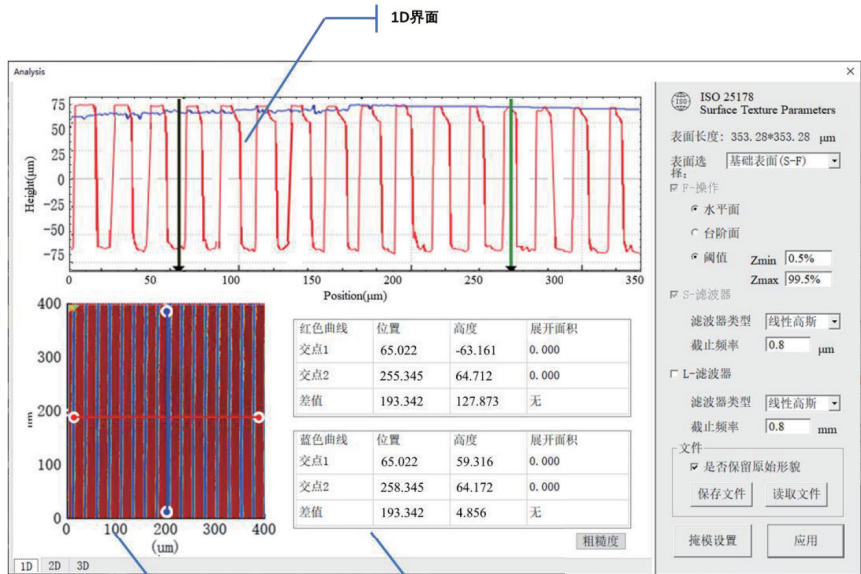
2D界面
