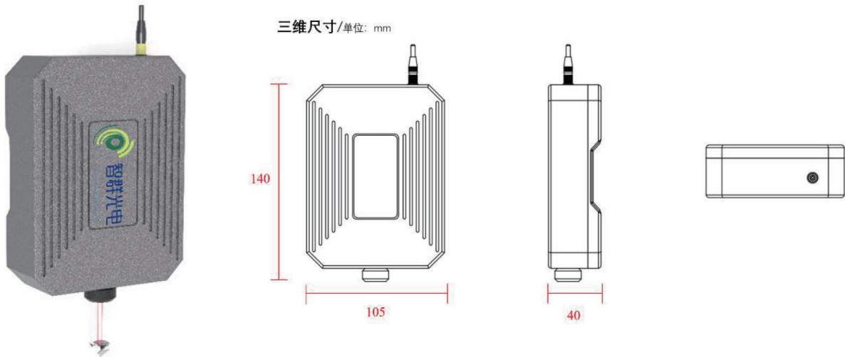
型号: IS-MD-01
